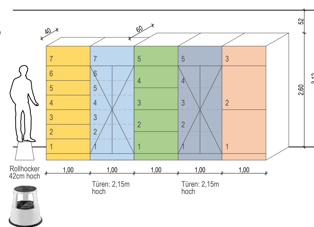
Legende Lagerregale
